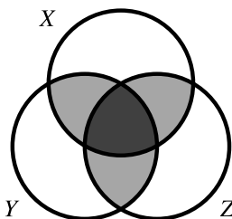
Fig. 5.1. Enumerating X \cup Y \cup Z
